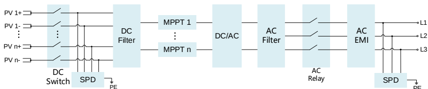
Stromlaufplan
