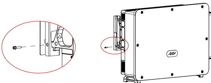
Wechselrichter befestigen
