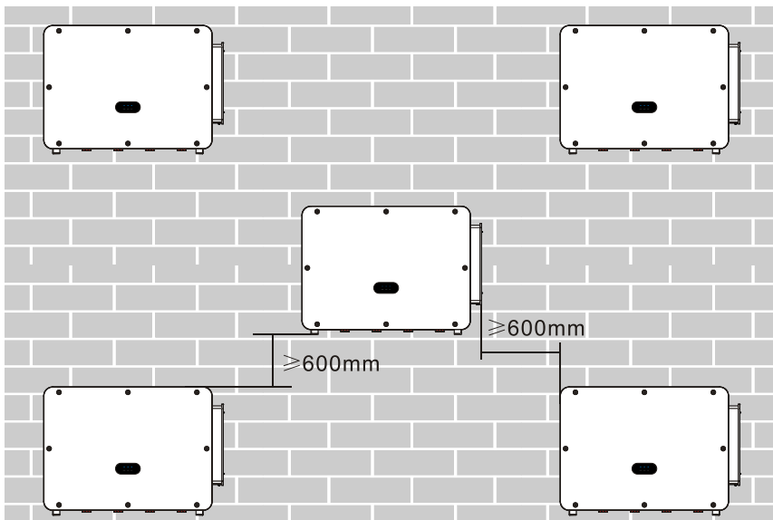
b) Nicht empfohlene Installationsmethode
