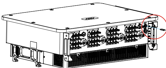
Schema des USB-Zugangs
