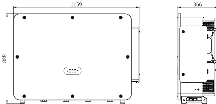
Abmessungen der Vorderansicht und der linken Ansicht des Produkts
