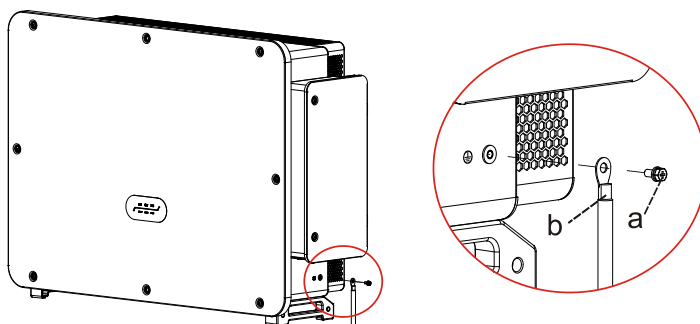
A. M8-Sechskantschraube B. Erdungskabel
