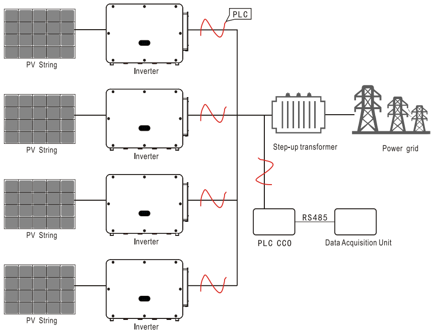
Multi-Wechselrichter-Überwachungssystem
