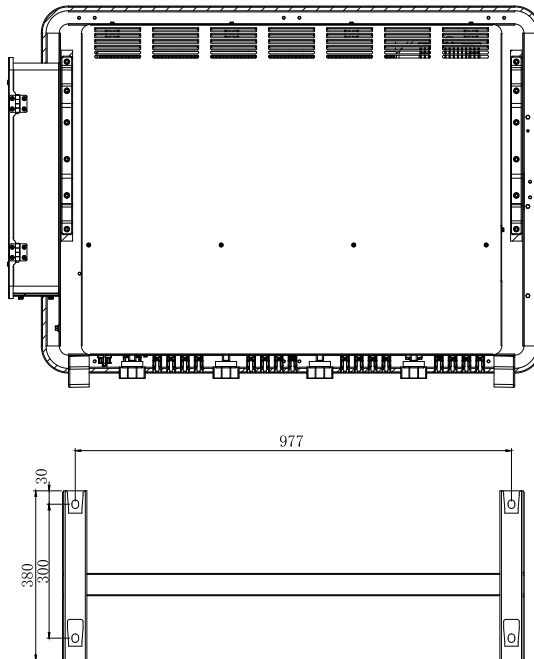
Abmessungen der Vorderansicht und der linken Ansicht des Produkts
