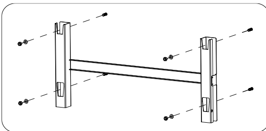
Wandhalterung installieren
