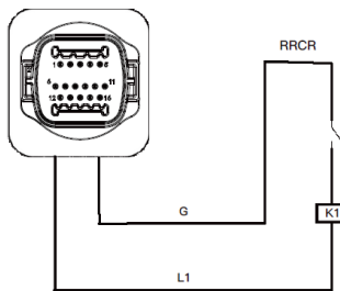
Wechselrichter - RRCR-Anschluss
