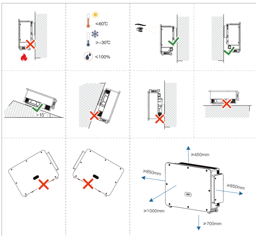
Auswahl des Installationsort
