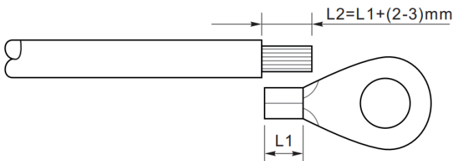
Anleitung für den Erdungsanschluss (1)
